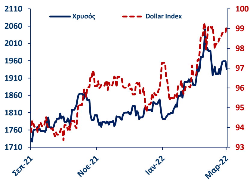
ΧΡΥΣΟΣ (USD/OZ)
