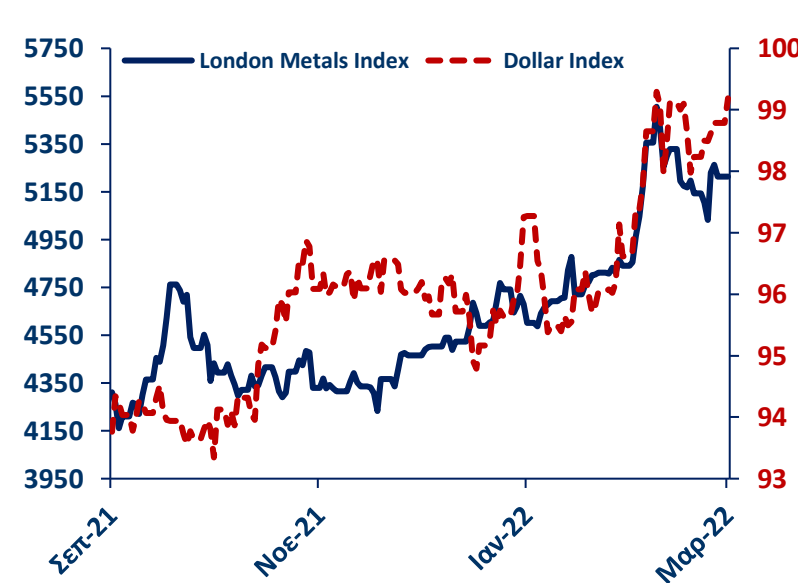
ΔΕΙΚΤΗΣ ΜΕΤΑΛΛΩΝ
