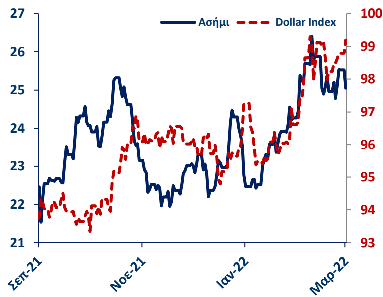
ΑΣΗΜΙ (USD/OZ)
